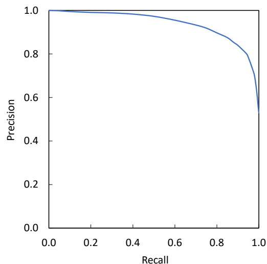
図6 Precision-Recall曲線
