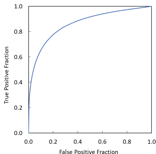
図5 ROC曲線
